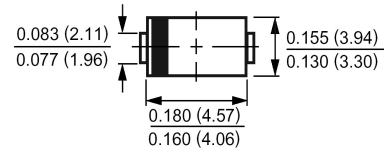
DO214-AA(SMB)
