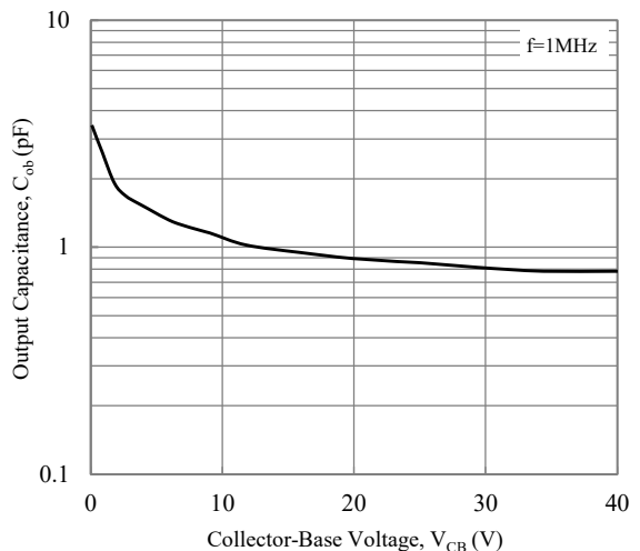
Fig. 6 Output Capacitance
