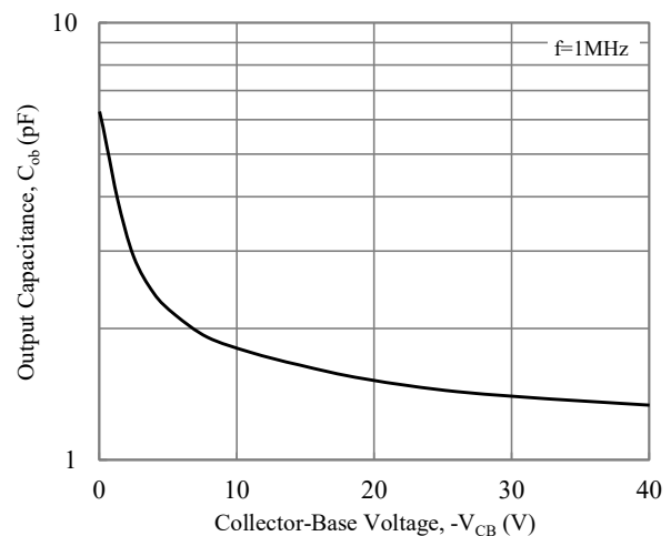
Fig. 6 Output Capacitance
